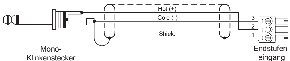
Anschlusskabel für Geräte mit unsymmetrischen Ausgängen
