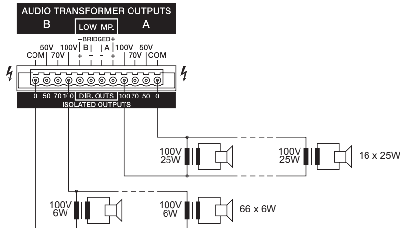
Exemple de configuration : PCL 1240T avec haut-parleur de 100V connecté. Charges de travail maximum avec haut-parleurs de 25W/100V et 6W/100V.
