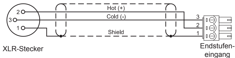
Anschlusskabel für Geräte mit symmetrischen XLR-Ausgängen
