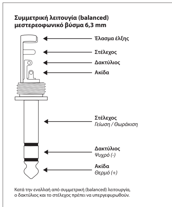
Εικ. 8.1: 6,3 χιλ. βύσμα υποδοχής στέρεο
