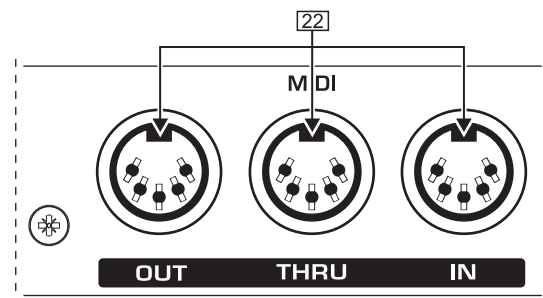
Εικ. 3.5: Υποδοχές σύνδεσης MIDI του FBQ2496
