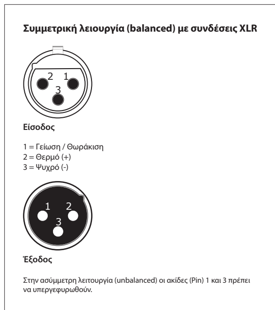
Εικ. 8.2: Βύσμα XLR
