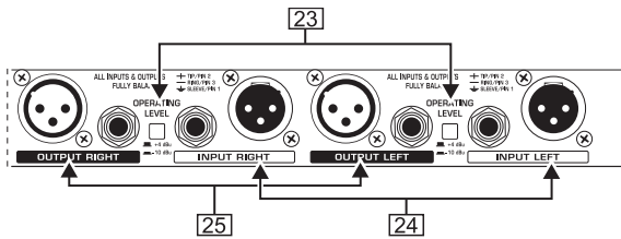
Εικ. 3.6: Συνδέσεις στην όπισθεν πλευρά του FBQ2496
