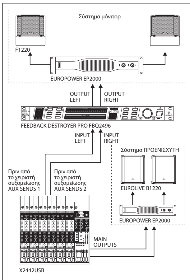
Εικ. 5.1: Χρήση του FBQ2496 στην οδό μόνιτορ
