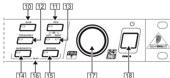
Εικ. 3.3: Στοιχεία χειρισμού στην δεξιά πλευρά του FBQ2496
