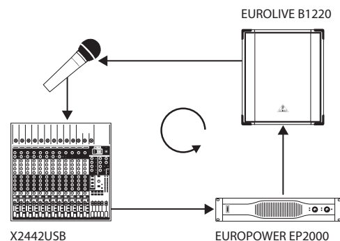
Εικ. 2.1: Δημιουργία ενός βρόχου ανάδρασης
